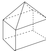
Figura 1: Alcuni poliedri.
