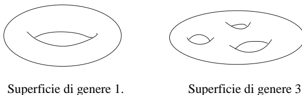
Figura 11: Superfici orientabili.
