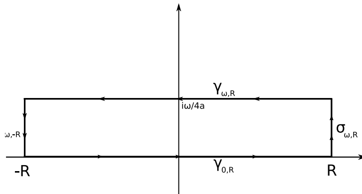
Figura 6.1: curve utilizzate nel calcolo della trasformata di e^{-at^2}
